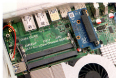
● 兩條SO-DIMM記憶體插槽位於黑色的2.5吋硬碟架下方。
